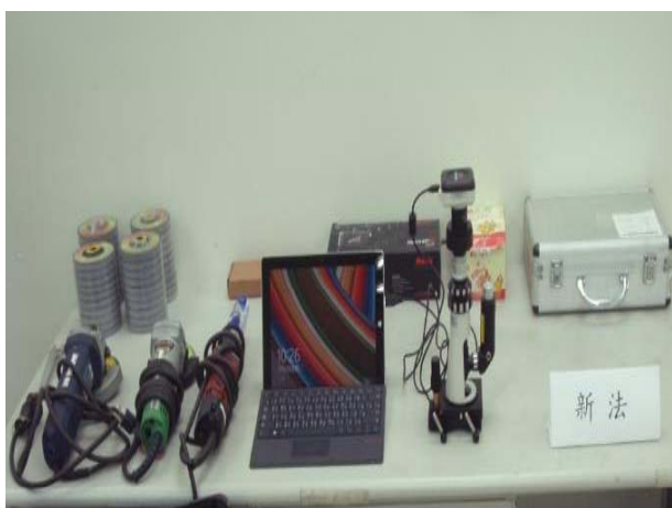
現場金相分析設備
