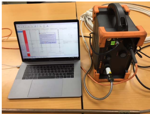
遠/近場渦電流檢測系統
